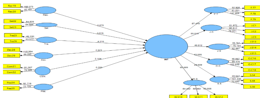
شکل ۲. خروجی آماره تی
