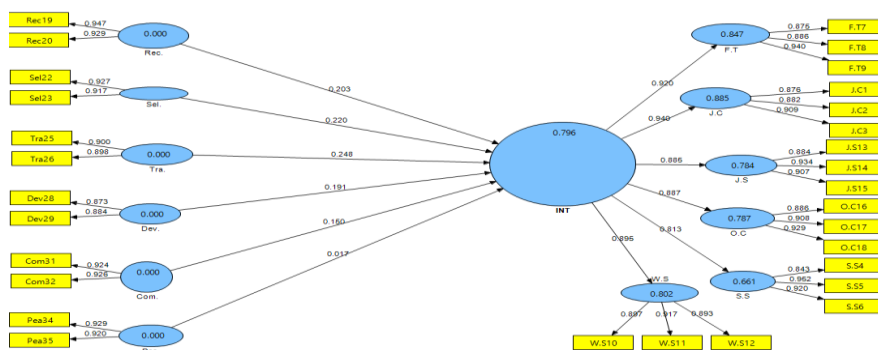
شکل ۱. خروجی ضریب مسیر استاندارد
